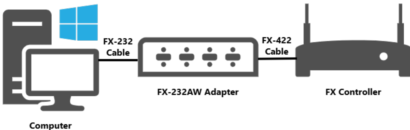
Conexão de um equipamento Melsec-FX via porta serial
