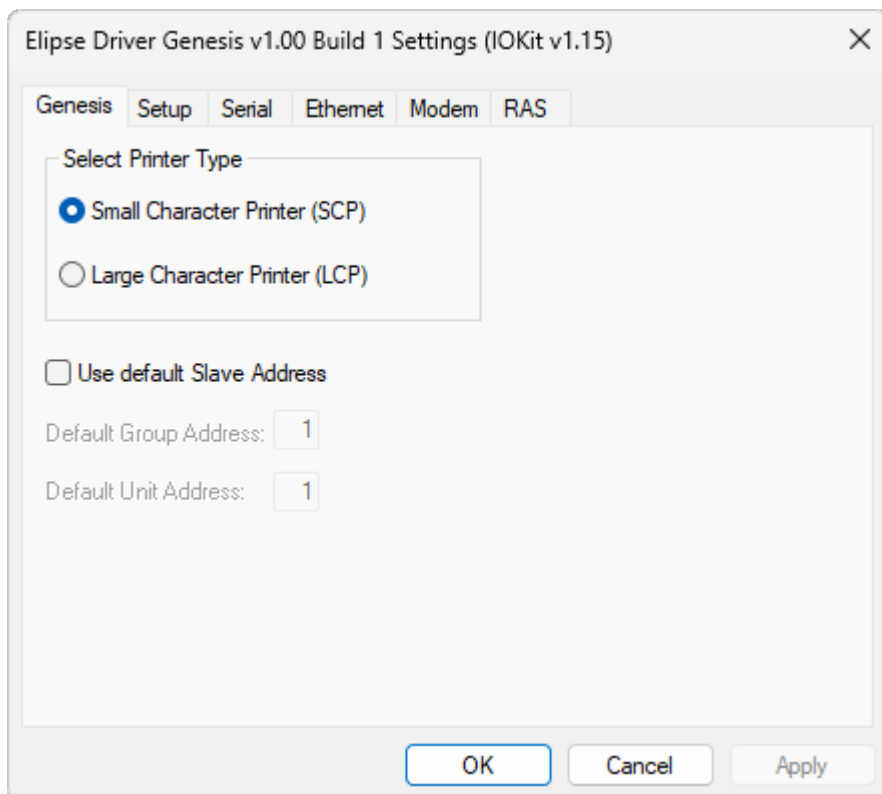
Genesis tab
