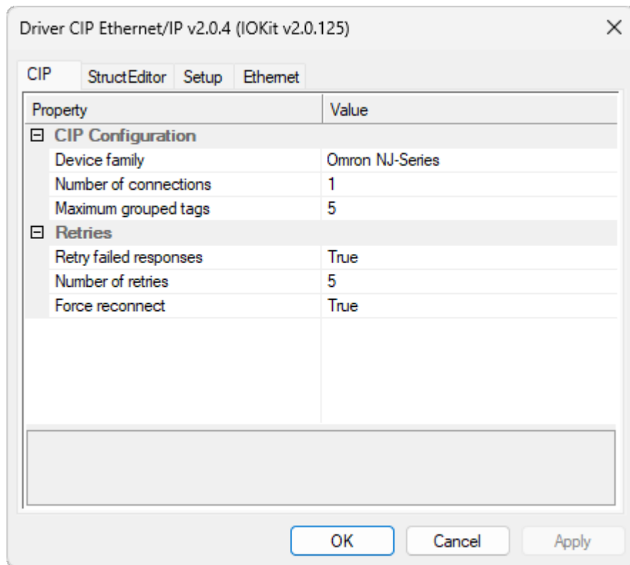
CIP tab
